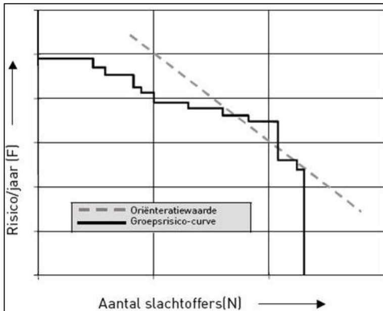
Figuur 1 : Groepsrisicocurve
